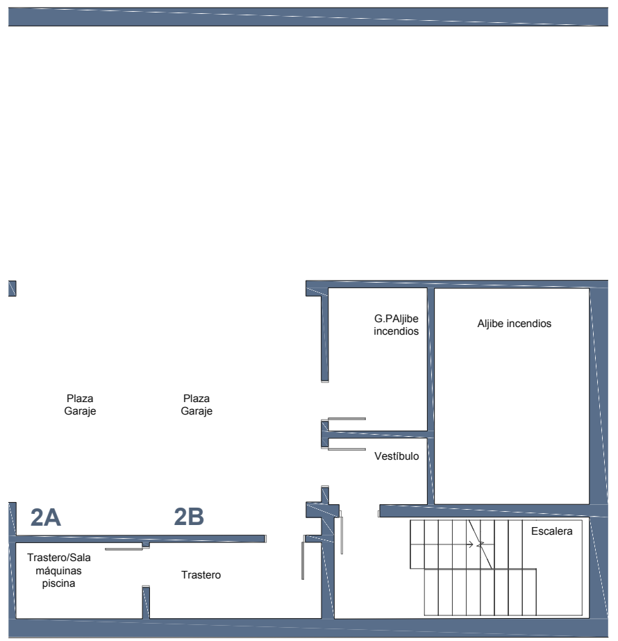
Basement | Sótano | Keller
