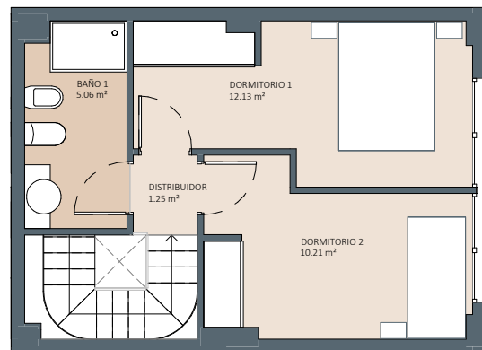
PLANTA ALTA
