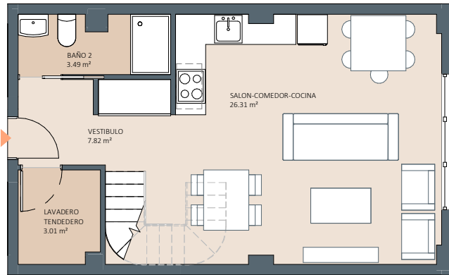
PLANTA BAJA
