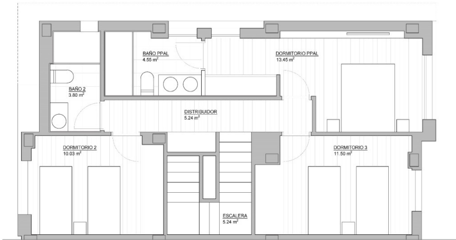
PLANTA PRIMERA
