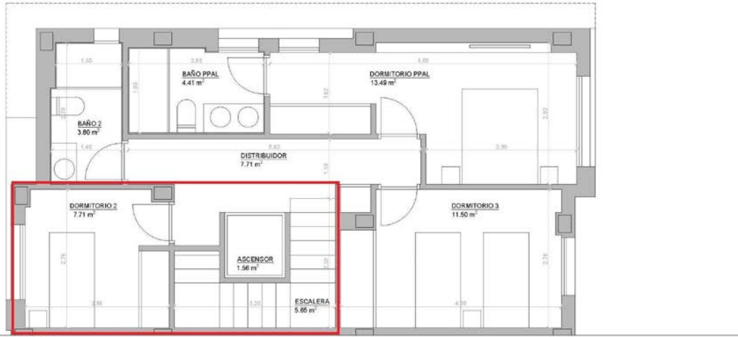
PLANTA PRIMERA
