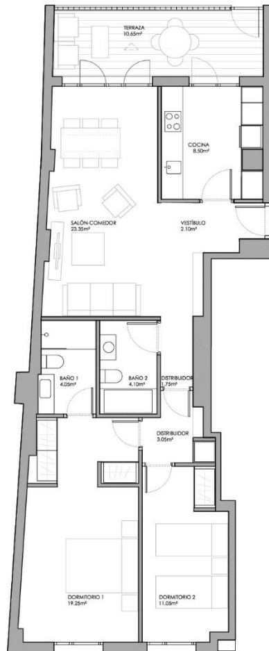
VT A1 - 2 Dormitorios Planta baja (1 Uds)
