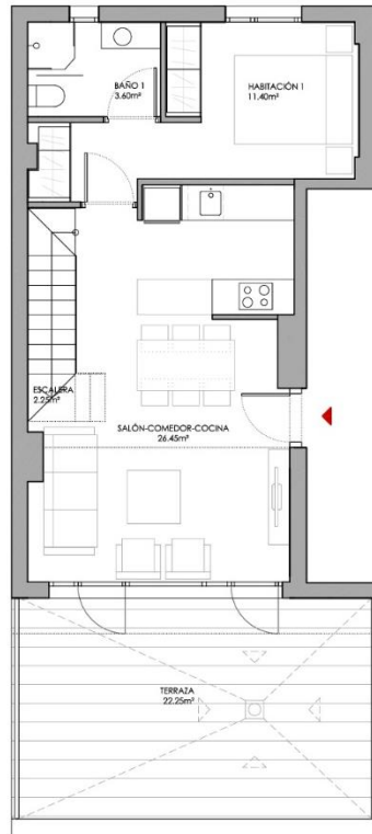
VT D3 - 1 Dormitor+Desván Planta ático (1 Uds)
