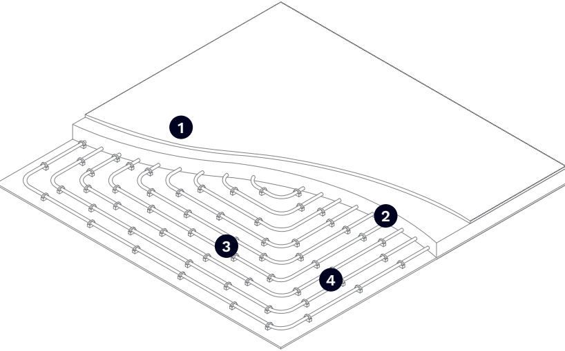
Suelo radiante
