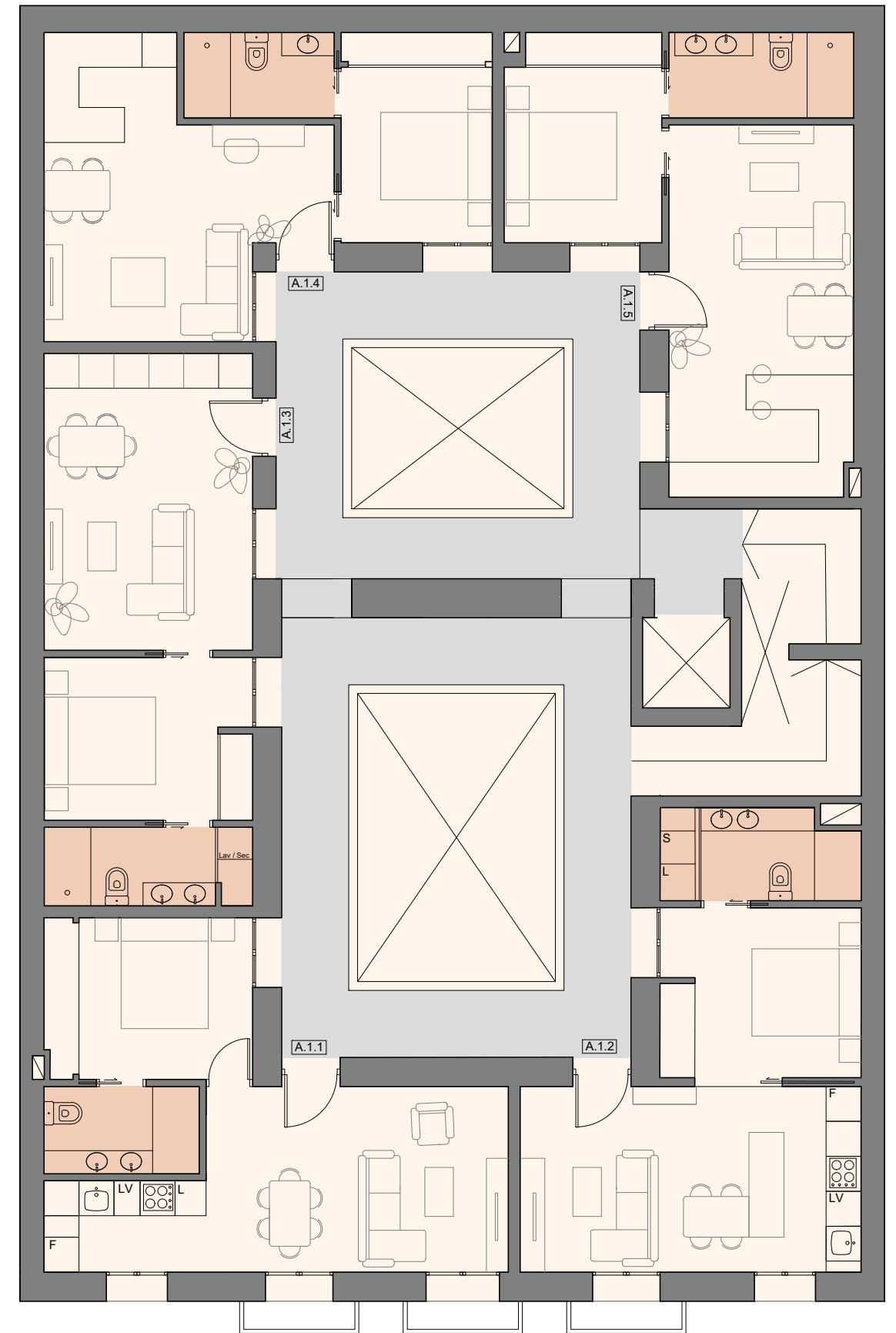
PLANTA PRIMERA
