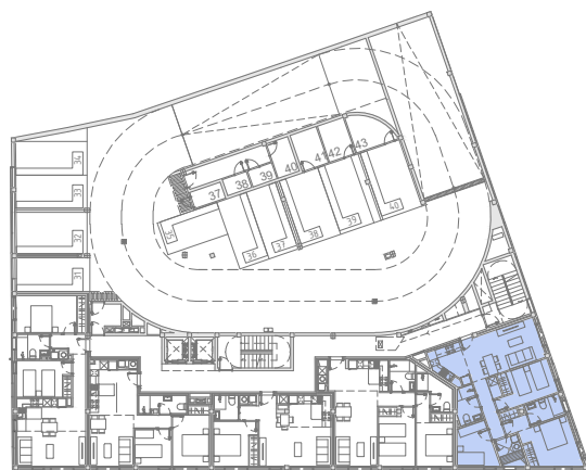
PLANTA SEGUNDA | 2
