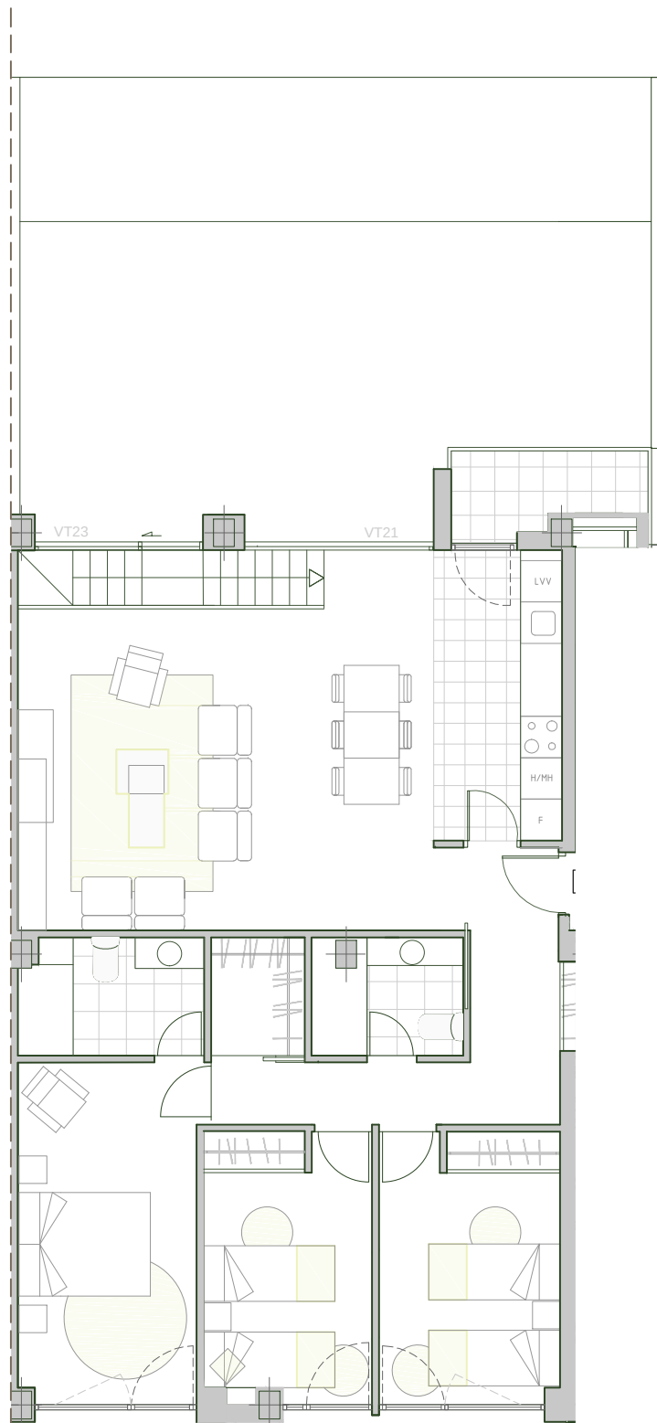
PLANTA ACCESO
